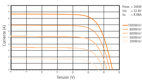
PCA200 – Curvas de salida nominales con 1000 W/m 2
