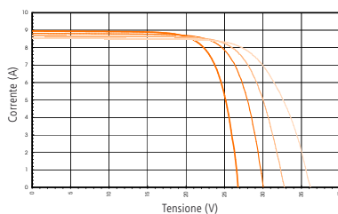
PCA 200 – curve di potenza nominale a 1000 W/m 2
