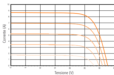
PCA 200 – curve di potenza nominale a 1000 W/m 2
